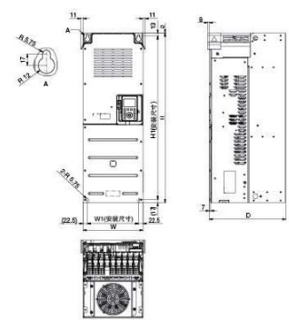
A6型外形图
