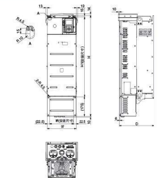
A5型外形图
