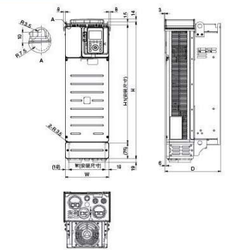
A4型外形图
