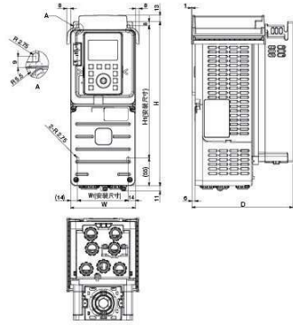
A1 型外形图
