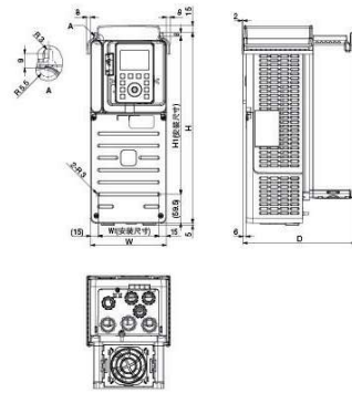
A2型外形图
