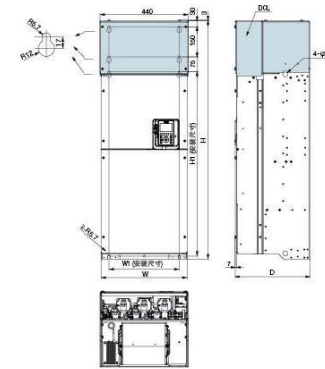
A7型外形图
