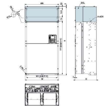
A8型外形图
