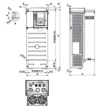
A3型外形图
