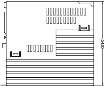
图 9-1 A 结构安装尺寸图
