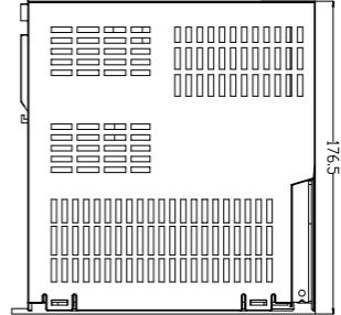
图 9-2 B 结构安装尺寸图
